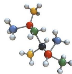
Amino acidi
